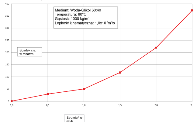
Spadek ciśnienia dla DN 16 dla kolanka 90°, R30
