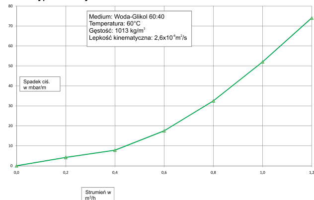
Spadek ciśnienia dla DN 16 stanie wyprostowanym
